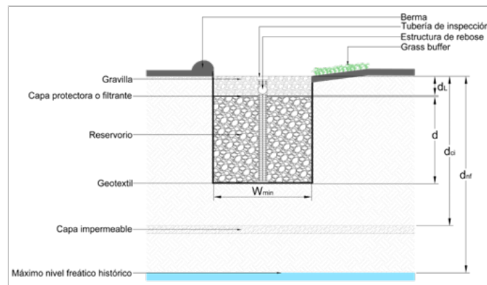
Figura 9. Sección transversal de la estructura - Zanjas de Infiltración. Fuente: Hoja de cálculo de zanjas de infiltración, Anexo NS-166 EAAB-Norma Técnica 1
